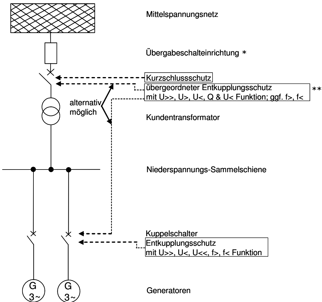
Bild C.5: An das Mittelspannungsnetz angeschlossene Erzeugungsanlage mit Leistungsschalter und mehreren Erzeugungseinheiten ohne Inselbetriebmöglichkeit
